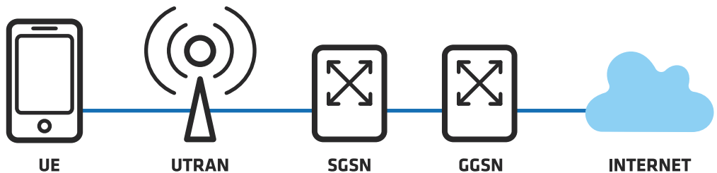
FIGURA 1: ARQUITECTURA GPRS BÁSICA
