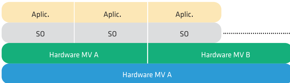
FIGURA 1: EMULACIÓN
